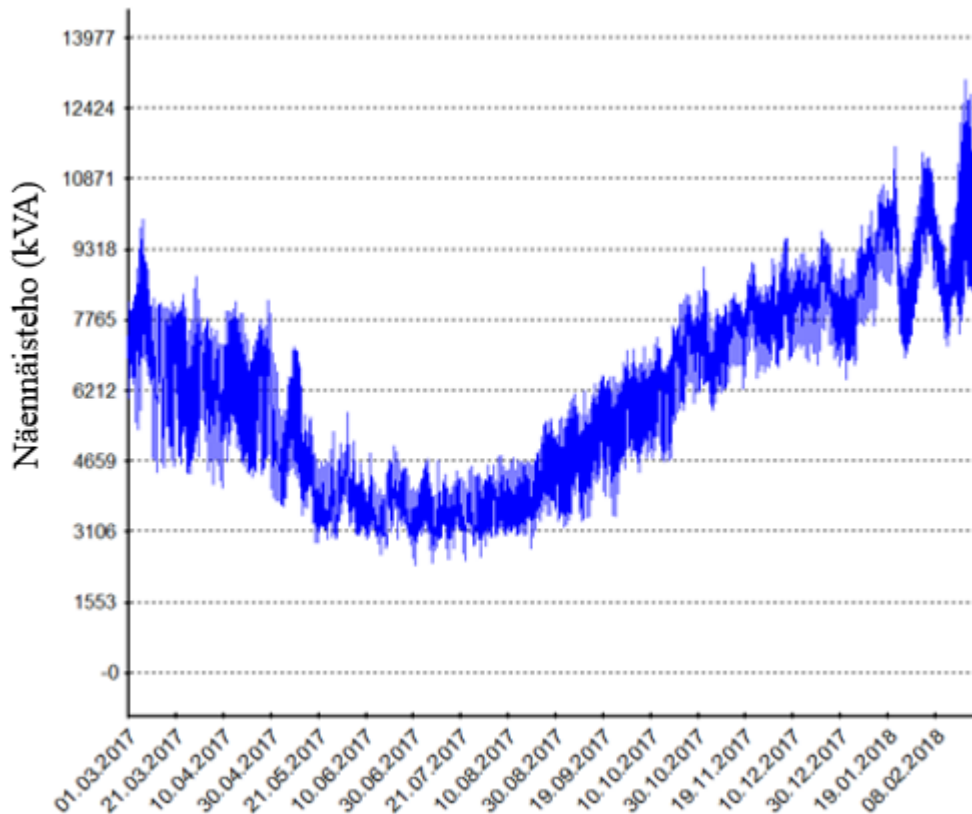
Kuva 5.1 Kangasalan Herttualan sähköaseman PT2 tehokuvaaja ajanjaksolta 01.03.2017–28.02.2018
